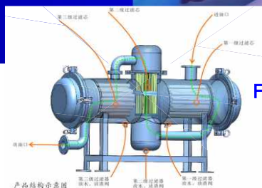
产品结构示意图
