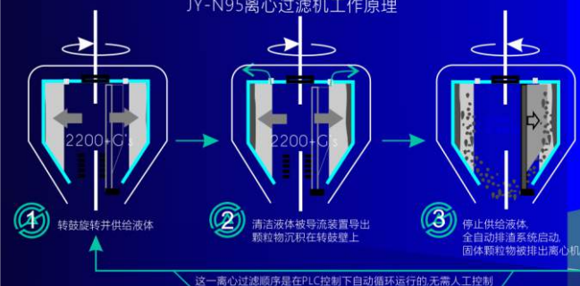
JY-N95离心过滤机工作原理
